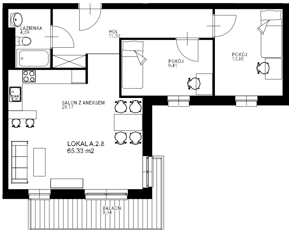
RZUT MIESZKANIA SKALA 1:100
