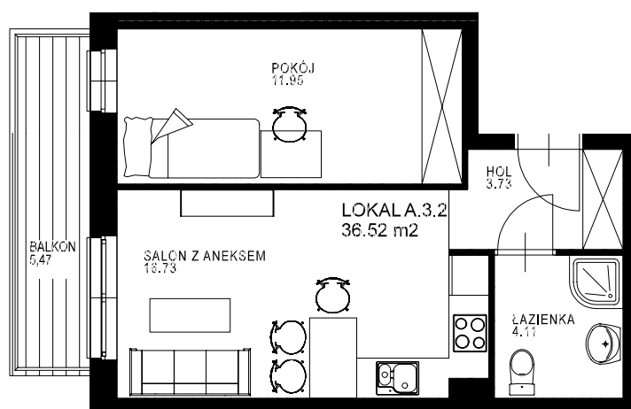
RZUT MIESZKANIA SKALA 1:100
