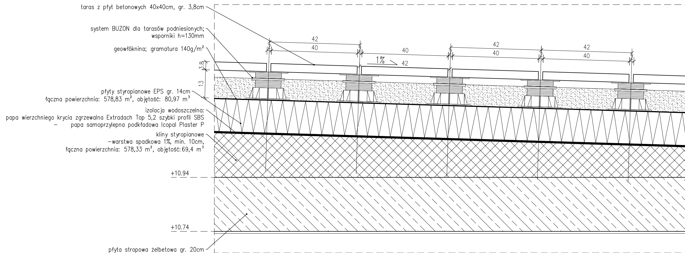
TARAS NA DACHU; 1:10 PŁYTY BETONOWE 40x40x3.8 SYSTEM PODŁOGI PODNIESIONEJ BUZON
